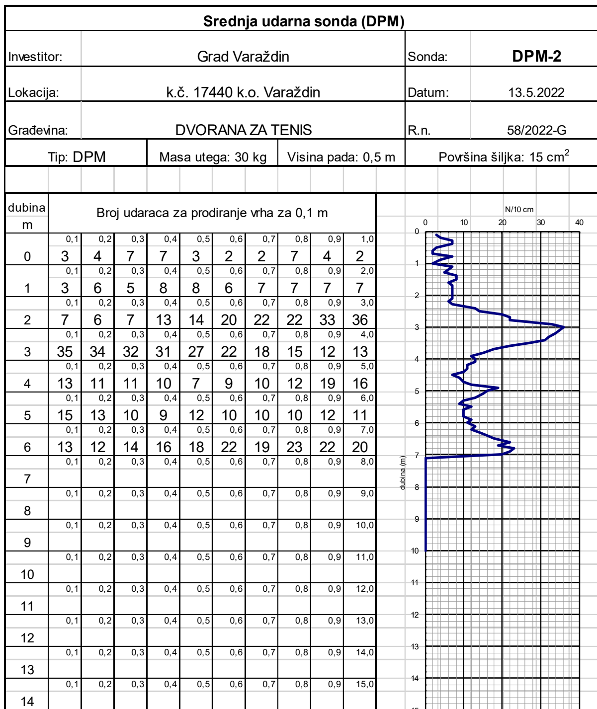
Slika 6. Dijagram ispitivanja srednjom udarnom sondom DPM -2
